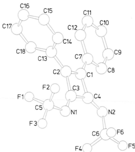
Abb. 1. Molekülstruktur von 1,2-Diphenyl-3,4-bis(trifluormethylimino)cyclobuten (SCHAKAL-Zeichnung [11]).
