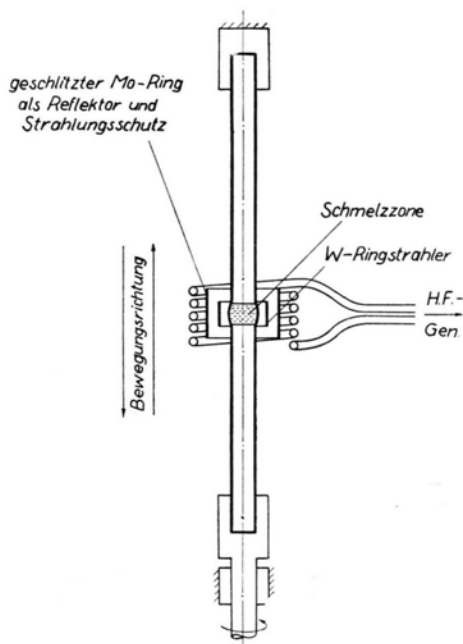
Abb. 1. Tiegelreies Schmelzen in senkrechter Anordnung.
